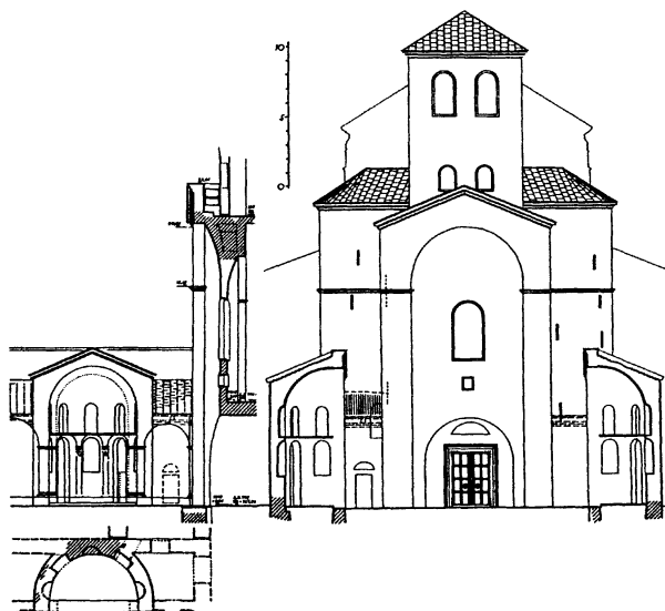
Az aacheni palota metszetrajzai
