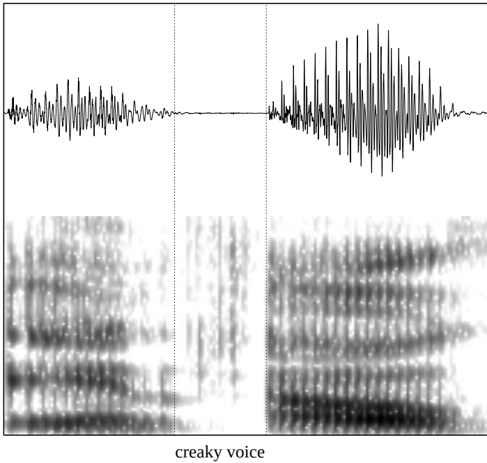
Abbildung 22: creaky voice an der Wortgrenze in Augsburg auf einem Breitbandsonagramm
