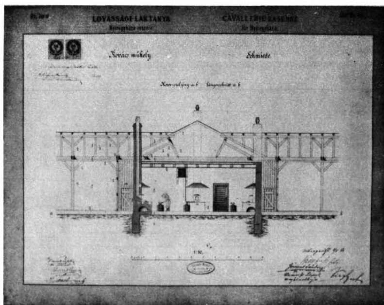
A kovácműhely metszete
