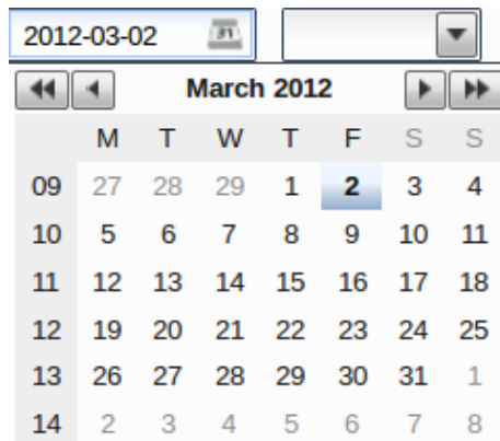
Dátumválasztó widget
