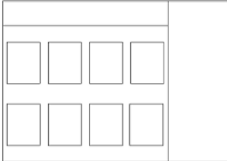
A képernyőterv ...
